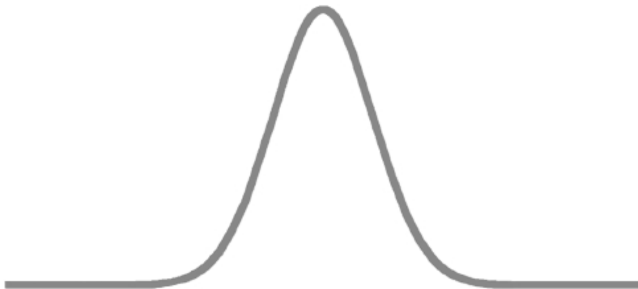
FIGURA 14. Uma versão mais abstrata: curva de Platão. Um número infinito de lances da moeda.
