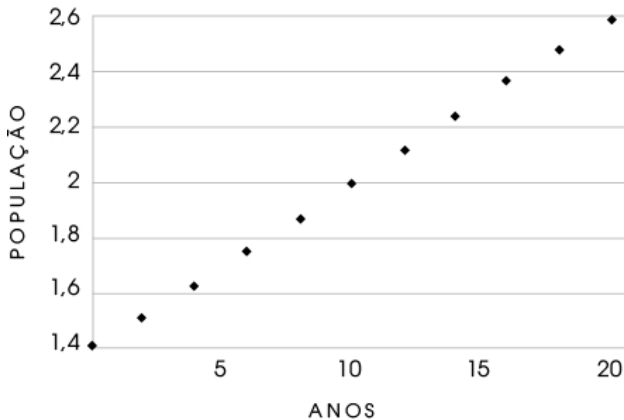
FIGURA 6. Uma série de uma população de bactérias aparentemente em crescimento (ou de um histórico de vendas, ou de qualquer variável observada ao longo do tempo — como a alimentação total do peru no capítulo 4).
