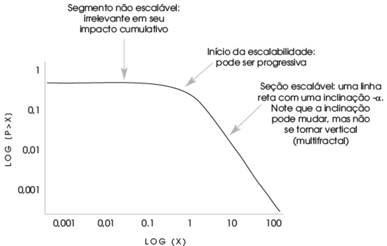
FIGURA 19. Distribuição típica com caudas de lei de potência (aqui uma distribuição T de Student).
