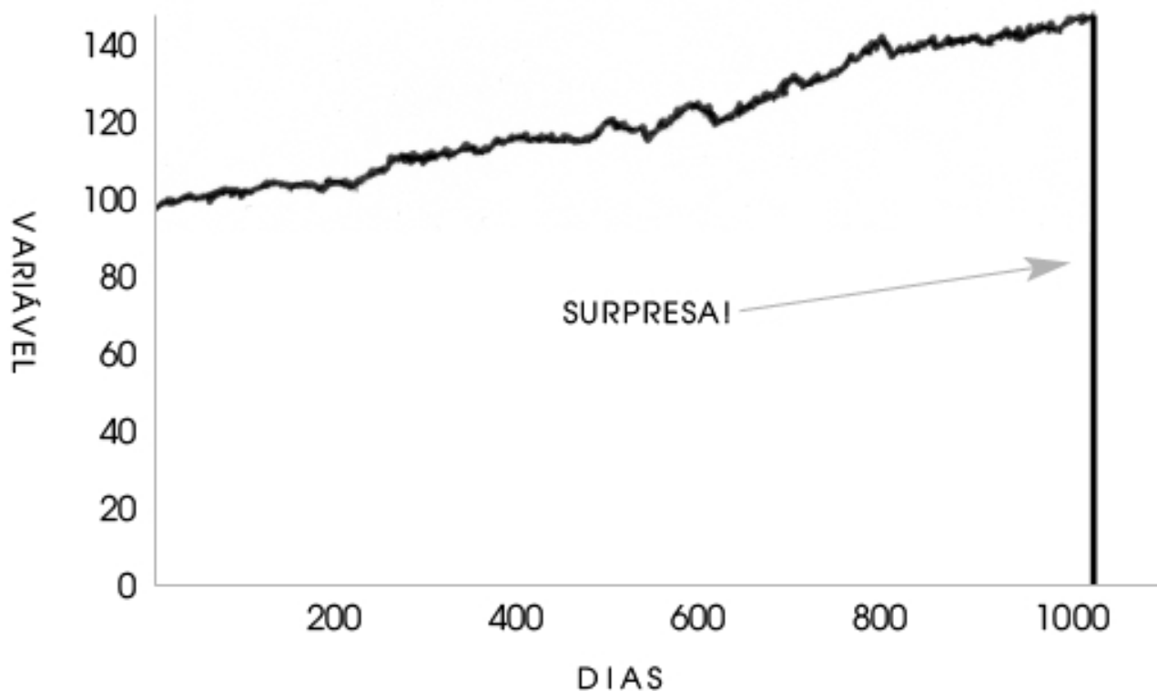
FIGURA 1. 1001 dias de história. Um peru antes e depois do Dia de Ação de Graças. A história de um processo de mais de mil dias de duração não diz nada sobre o que vai acontecer a seguir. Essa projeção ingênua do futuro com base no passado pode ser aplicada a qualquer coisa.
