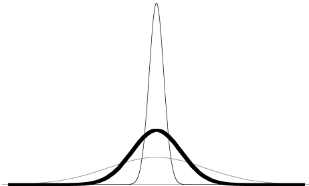
FIGURA 11. Como funciona a lei dos grandes números. No Mediocristão, à medida que o tamanho da amostragem aumenta, a média observada se apresenta com dispersão cada vez menor — como você pode ver, a distribuição será cada vez mais estreita. Em poucas palavras, na teoria estatística é assim que tudo funciona (ou deveria funcionar). No Mediocristão, a incerteza desaparece na média. Isso ilustra a banal “lei dos grandes números”.
