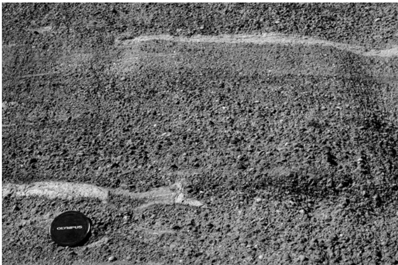
FIGURA 15. Aparentemente, uma tampa de lente de câmera caiu no chão.
