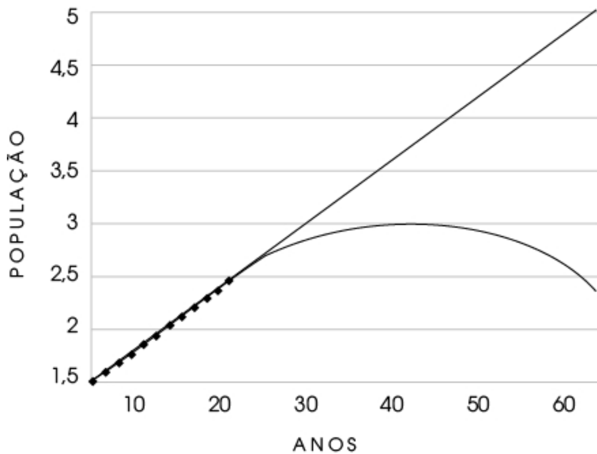
FIGURA 8. Observamos uma escala mais ampla. Ei, outros modelos também se encaixam muito bem.
