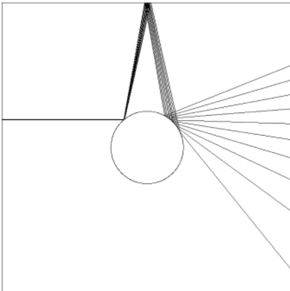
FIGURA 5. Precisão e previsão. Um dos leitores de um rascunho deste livro, David Cowan, graciosamente desenhou esta imagem que representa a dispersão, mostrando como, no segundo salto, as variações nas condições iniciais podem levar a resultados extremamente divergentes. À medida que a imprecisão inicial no ângulo é multiplicada, cada salto adicional será ainda mais ampliado. Isso causa um severo efeito multiplicativo em que o erro cresce de modo desproporcional.
