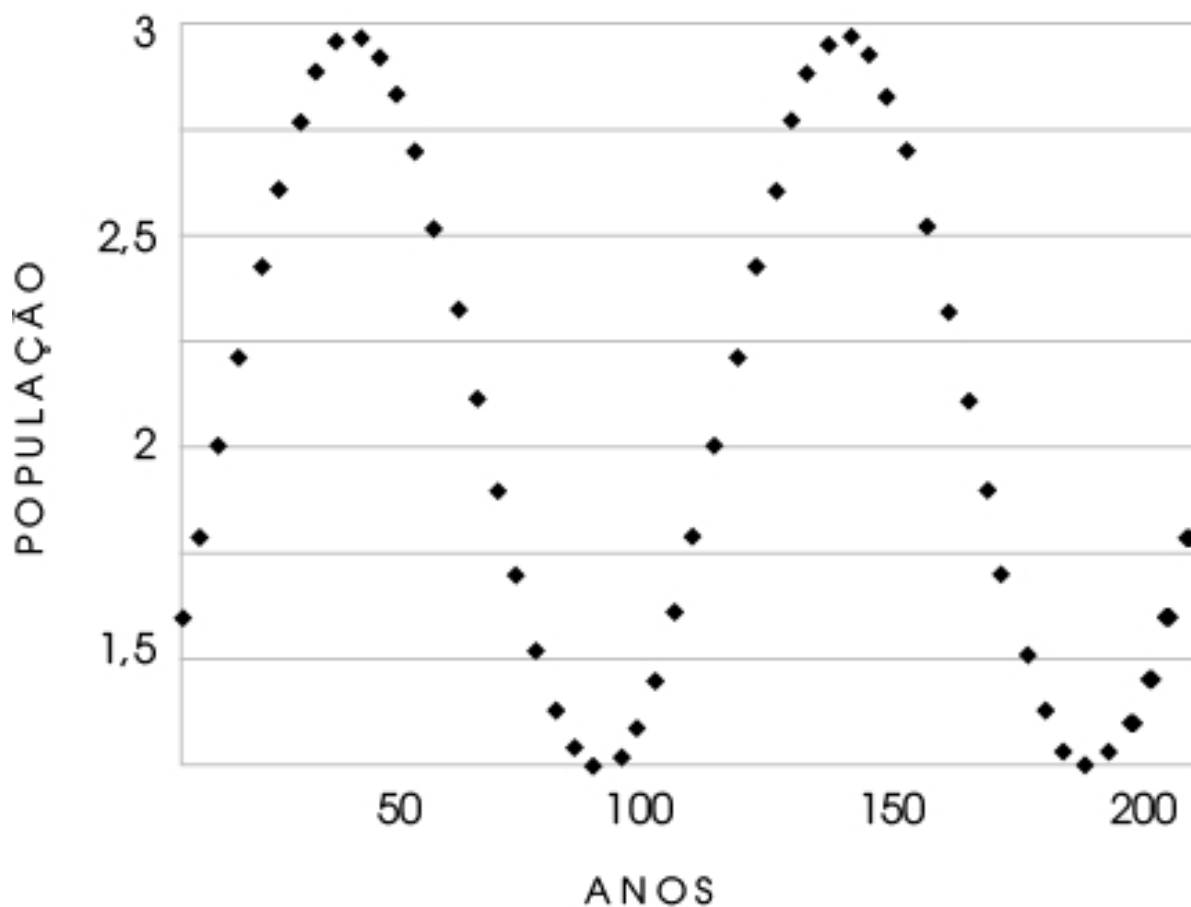
FIGURA 9. E o verdadeiro “processo gerador” é extremamente simples, mas não tinha nada a ver com um modelo linear! Algumas partes parecem ser lineares, e somos enganados ao extrapolar em uma linha direta. 7
