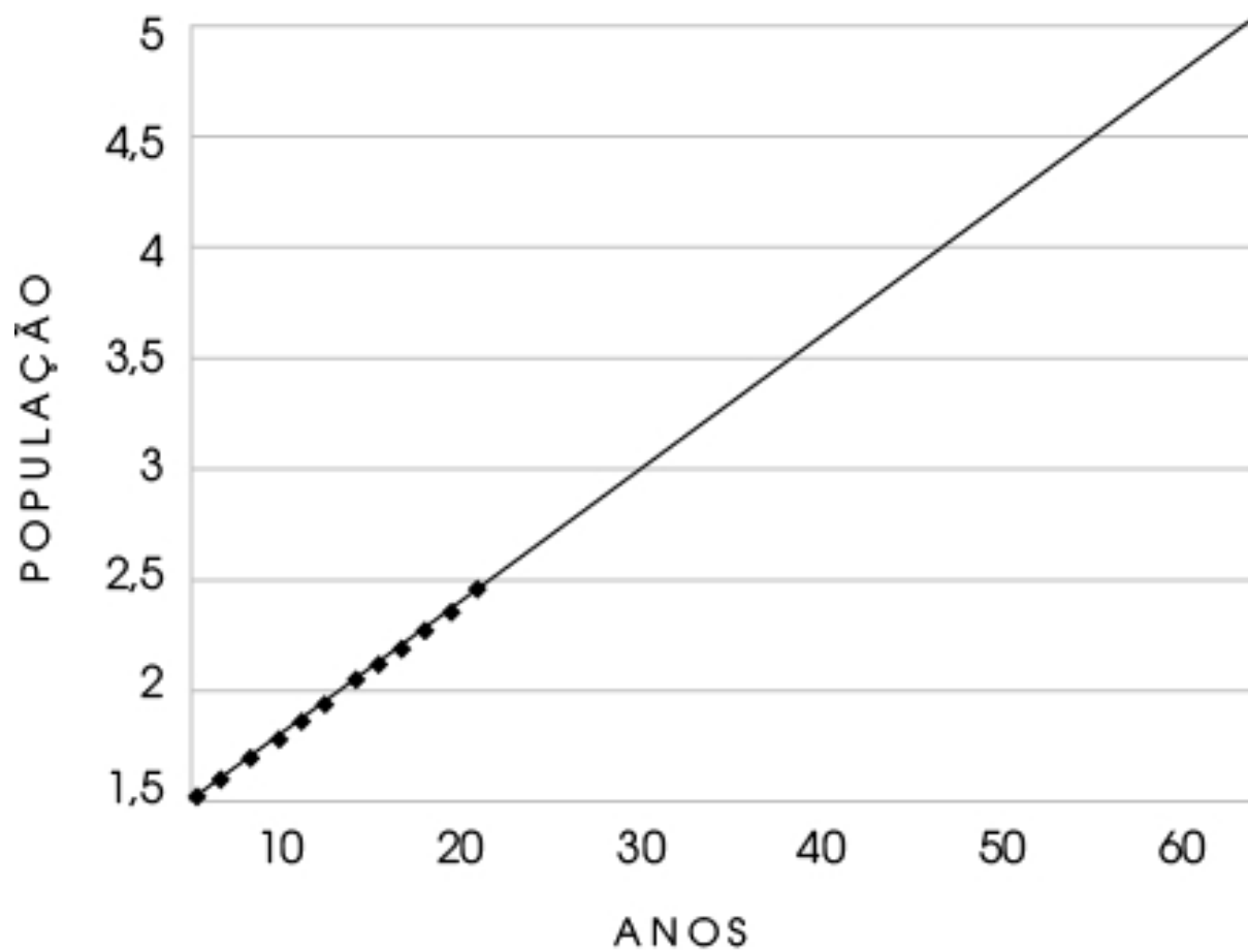
FIGURA 7. Fácil de se ajustar à tendência — há apenas um único modelo linear que se encaixa nos dados. Pode-se projetar uma continuação no futuro.
