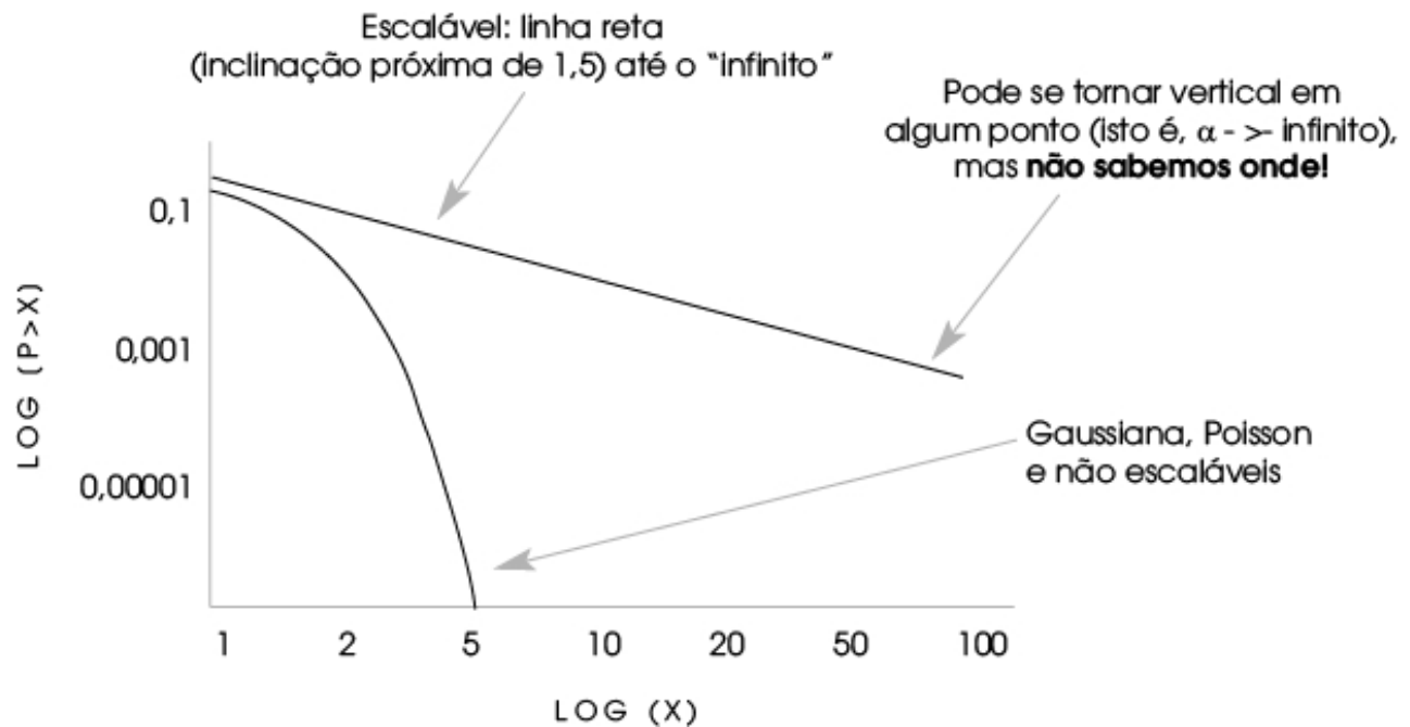
FIGURA 20. Os dois domínios exaustivos de atração: linha vertical ou linha reta com inclinações de infinito negativo ou a negativo constante. Note que, como as probabilidades precisam somar 1 (inclusive na França), não pode haver outras alternativas para as duas bacias, e é por isso que eu as limito a essas duas exclusivamente.
