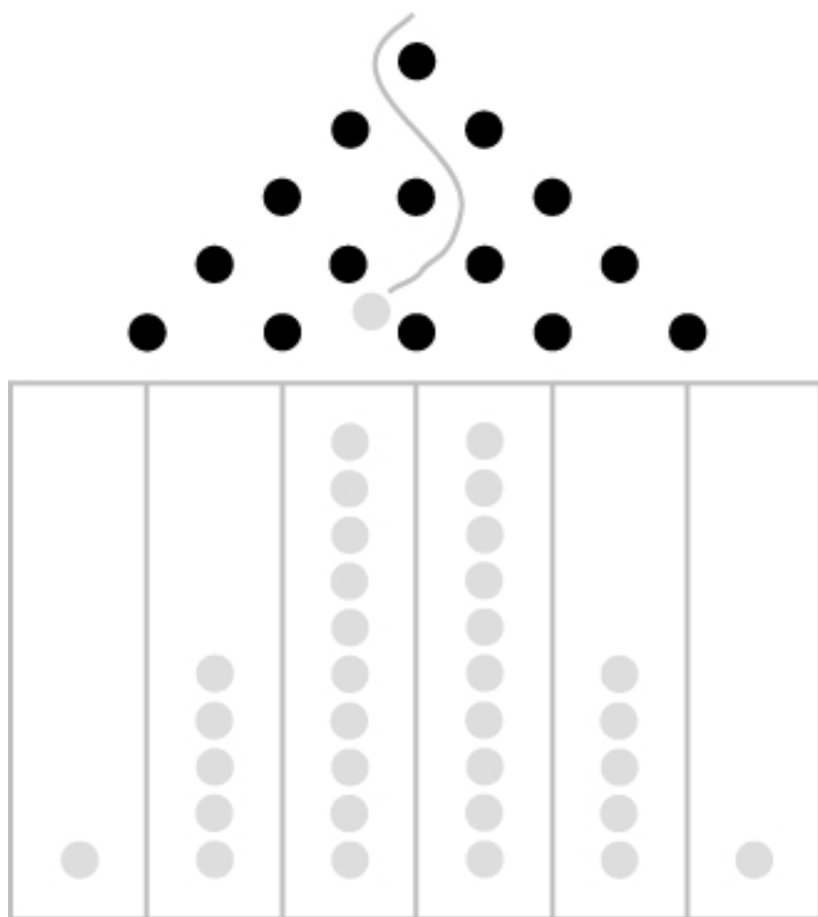
FIGURA 12. O quincunx (simplificado) — uma máquina de pinos. Solte bolas que, ao se chocarem contra um dos pinos distribuídos em forma de pirâmide e dispostos em intervalos iguais, caem aleatoriamente para a direita ou para a esquerda. A figura acima mostra o cenário hipotético mais provável, que se assemelha muito à curva em forma de sino (também conhecida como distribuição gaussiana). Cortesia de Alexander Taleb.
